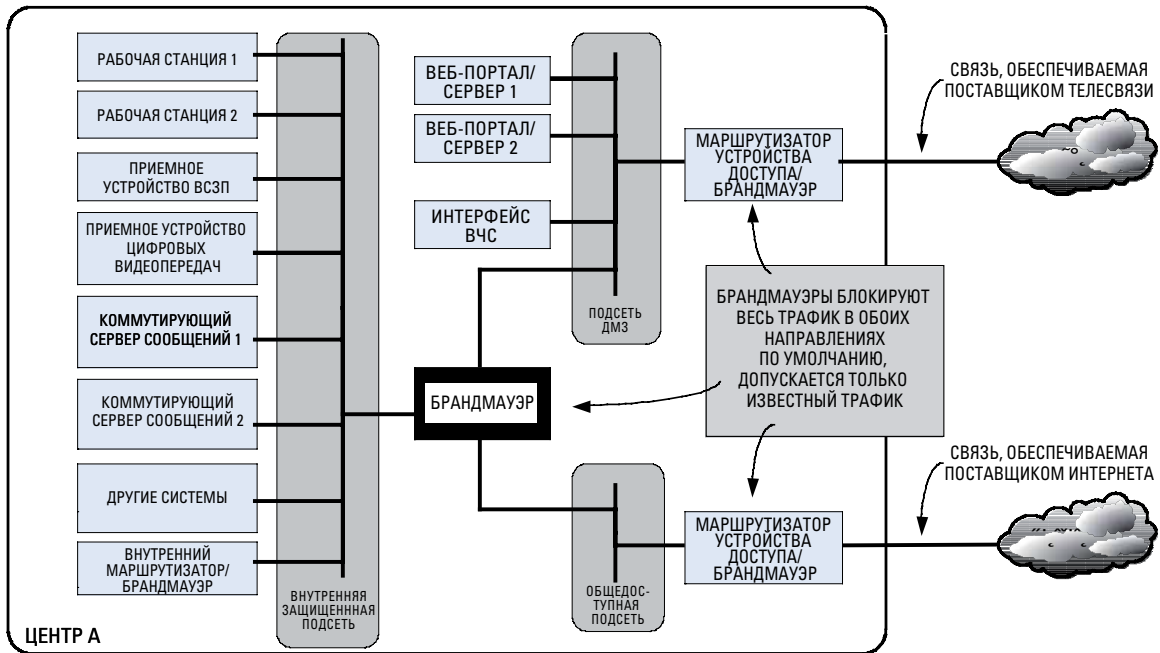
Рисунок 9. Топология сети ТСП/ИР в простом центре
