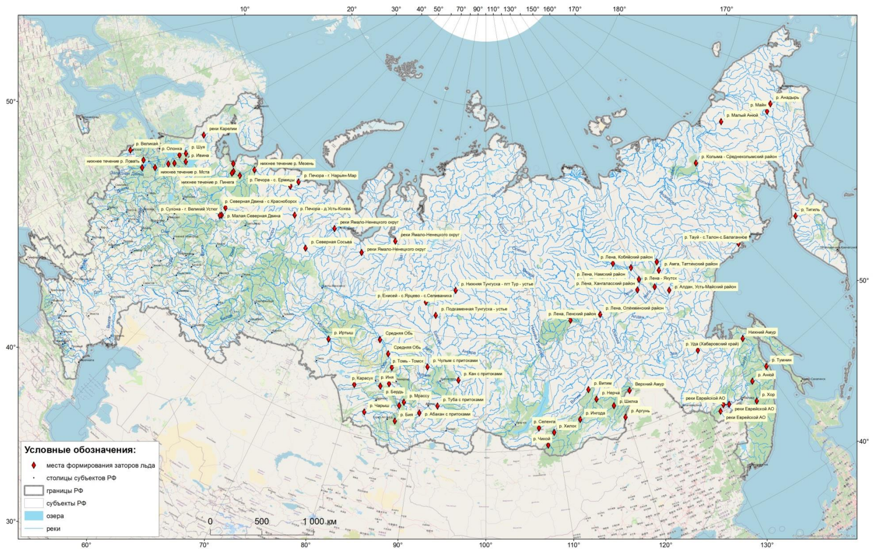
Рисунок 7. – Ожидаемые места формирования опасных затворов льда
