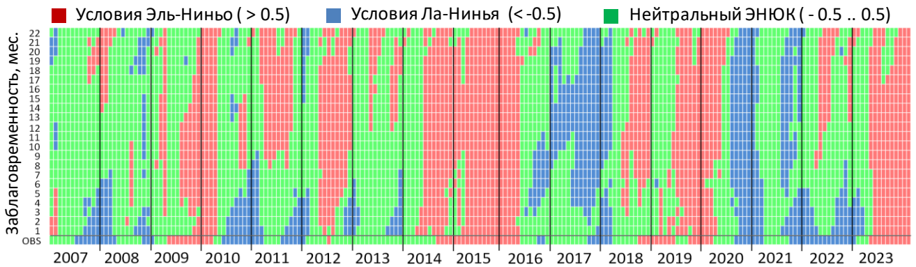
Рисунок Г.1 – Диаграмма состояния ЭНЮК за контрольный период 2007-2023 гг. по модельным расчетам с заблаговременностью до 22 месяцев на фоне данных реконструкции COBESST (на диаграмме ряд "OBS")
