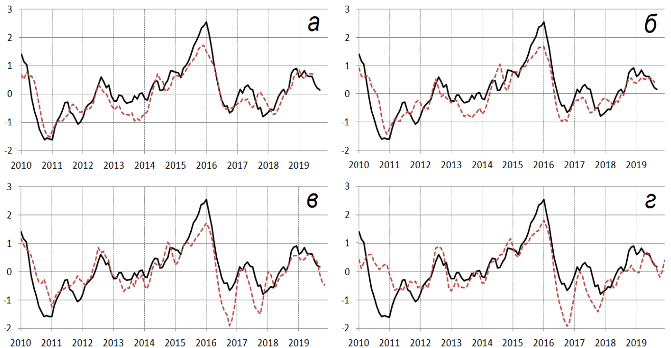
Рисунок 4.2 – Модельный индекс Niño 3.4 с заблаговременностью прогноза 3 (а), 5 (б), 7 (в) и 9 (г) месяцев (красный пунктир), и наблюдаемый Niño 3.4 (черная сплошная линия) за контрольный период 2010-2019
