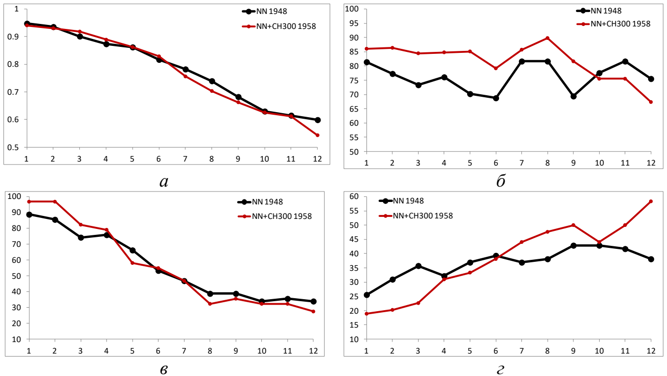
Рисунок В.2 – (а) – коэффициент корреляции за контрольный период (2007-2023) в зависимости от заблаговременности прогноза; (б) – повторяемость воспроизведения термических условий Эль-Ниньо; (в) – повторяемость воспроизведения термических условий Ла-Нинья; (г) – ошибочные термические условия Эль-Ниньо или Ла-Нинья. NN 1948 – обычная модель из параграфа 4.2; NN CH300 1958 – модель с учетом TCO300.
