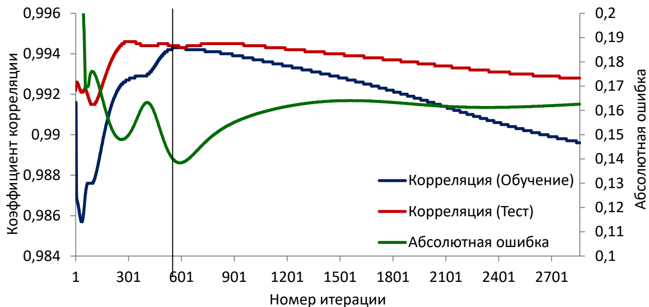
Рисунок 3.4 – Обучение и переобучение нейронной сети на примере искусственно созданных закономерностей с добавлением шума. Вертикальная линия обозначает момент максимума обучения.
