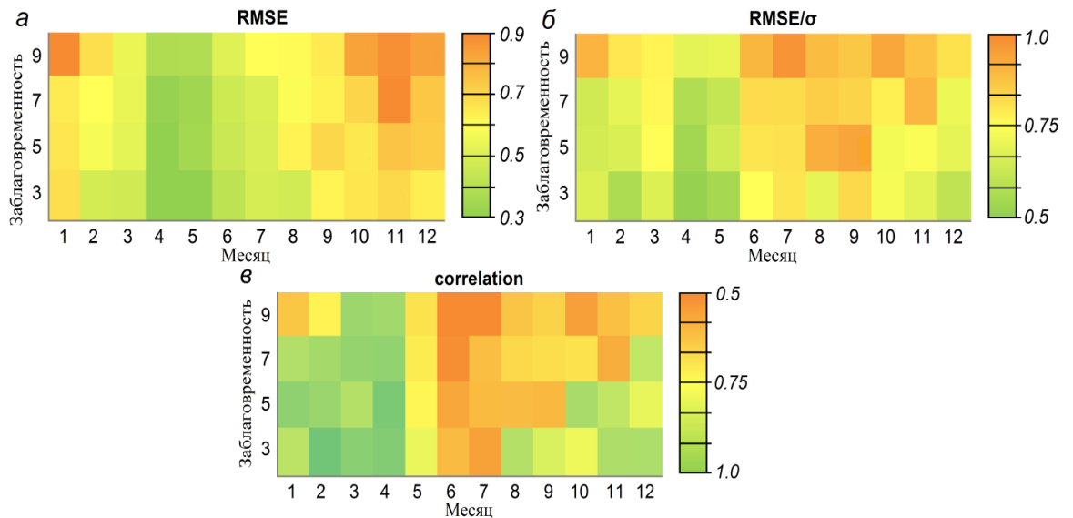
Рисунок 4.1 – Диаграммы зависимости RMSE (а), RMSE/\sigma (б) и коэффициента корреляции, r , (в) от прогнозируемого месяца и заблаговременности прогноза индекса Niño 3.4. (на основе t-критерия Стьюдента значимый r \geq 0.51 для 10 значений на уровне \alpha=0.01 )
