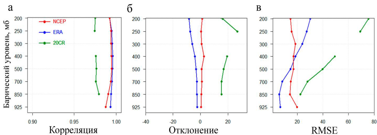
Рисунок 2.1 – Профили (а) – коэффициентов корреляции, (б) – средней ошибки и (в) – RMSE геопотенциала для реанализов NCEP/NCAR, ERA-Interim и 20CR в сравнении с данными аэрологического зондирования массива IGRA v2.1
