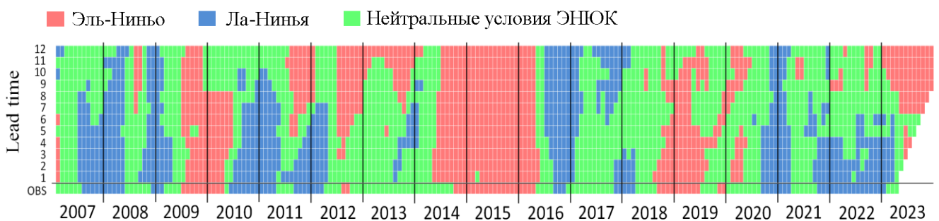
Рисунок В.3 – Состояние ЭНЮК за контрольный период 2007-2023 гг. по модельным расчетам с заблаговременностью до 12 месяцев на фоне данных реконструкции COBESST (на диаграмме ряд "OBS")
