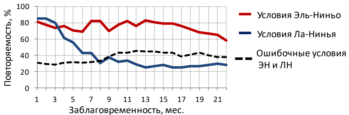
Рисунок Г.2 – Повторяемость воспроизведения термических условий Эль-Ниньо, Ла-Нинья и ошибочные условия Эль-Ниньо или Ла-Нинья
